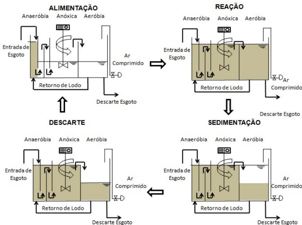
Figura 2: Fases que compõe o ciclo operacional
