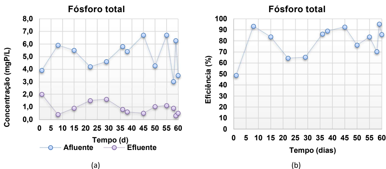
Figura 6: Série temporal (a) e eficiências (b) das concentrações de Fósforo Total obtidos durante o estudo.
