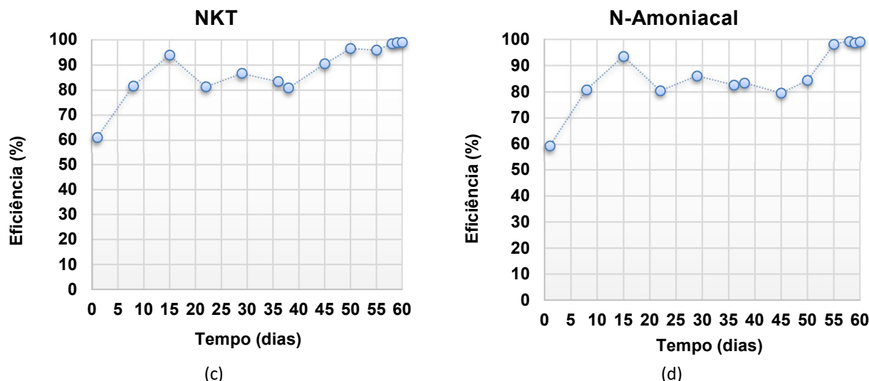
Figura 5: Série temporal (a/b) e eficiências (c/d) para concentrações de NKT e N-Amoniacal durante o estudo.
