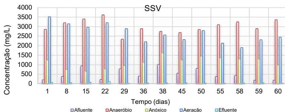
Figura 41: Série temporal das concentrações de SSV durante o estudo
