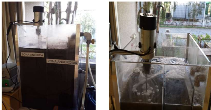
Figura 1: Sistema cíclico de lodo ativado
