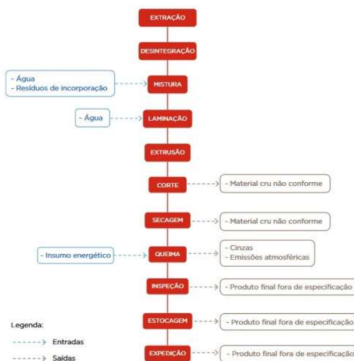
Figura 1: Fluxograma do processo produtivo. Fonte: Fiemg et al. (2013).
